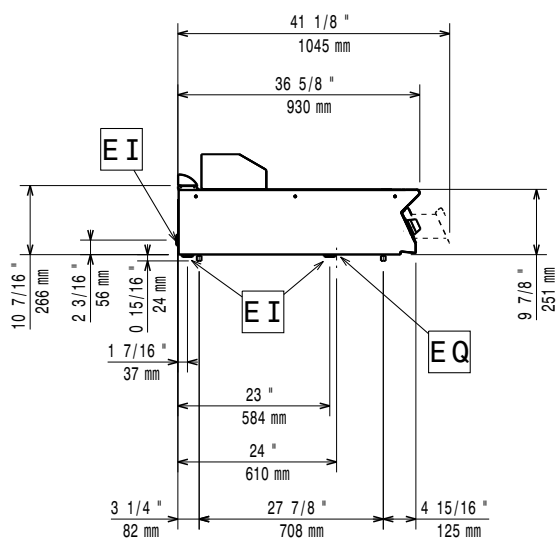
Oldalnézet
